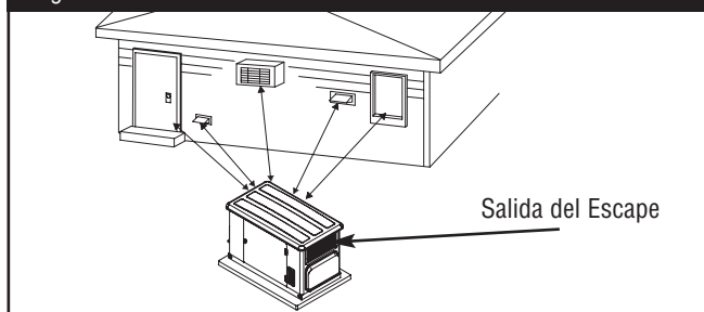
Figura 6 — Ubicación del Sistema de Generador de Doméstico
