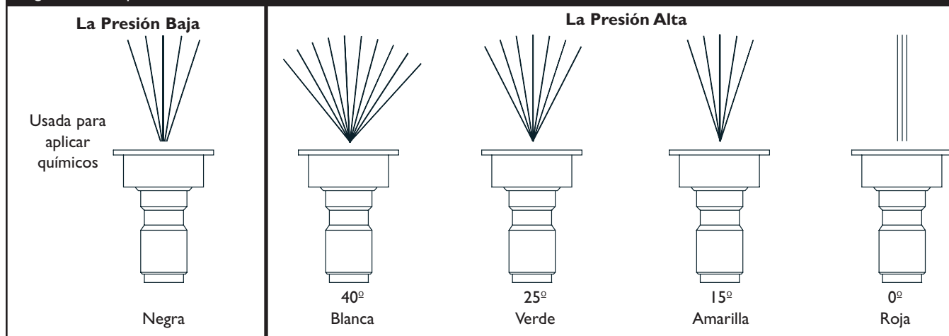
Figura 24 - Boquillas
