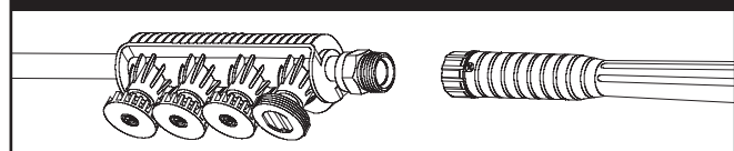
Figura 86 — Conecte la Extensión de la Lanza a la Pistola Rociadora
