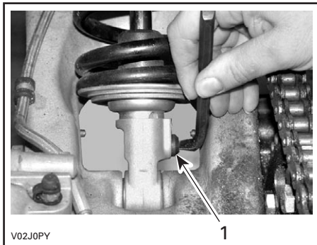
1. Adjuster
