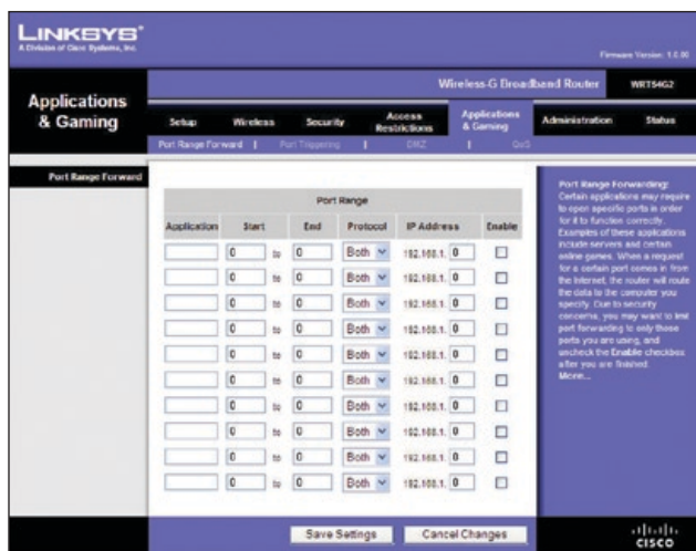
Aplicativos e Jogos - Port Range Forward (Encaminhamento de Intervalo de Portas)
