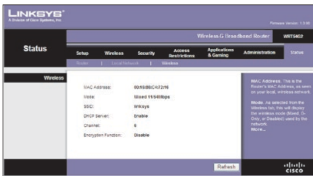
Status > Wireless (Estado > Inalámbrica)
