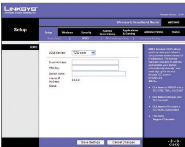
Configuração &gt; DDNS &gt; TZO
