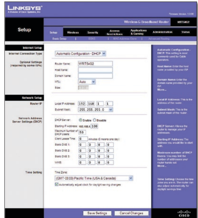
Setup > Basic Setup (Configuración > Configuración básica)
