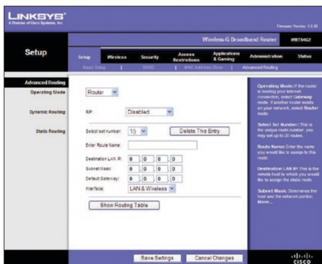
Setup > Advanced Routing (Configuração > Roteamento Avançado [Roteador])
