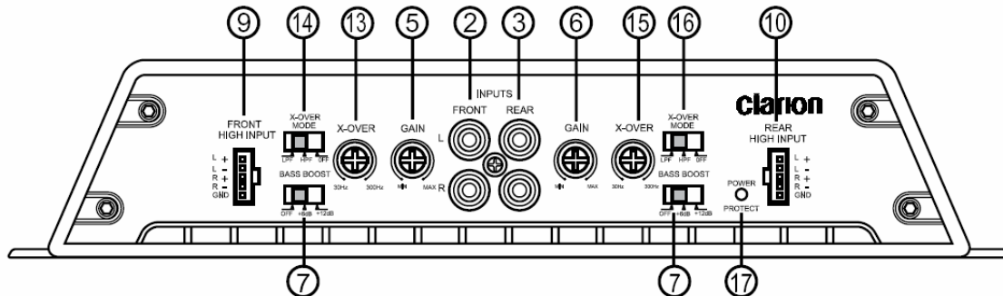
Модель APX4241E: ручки настройки и входные разъемы
