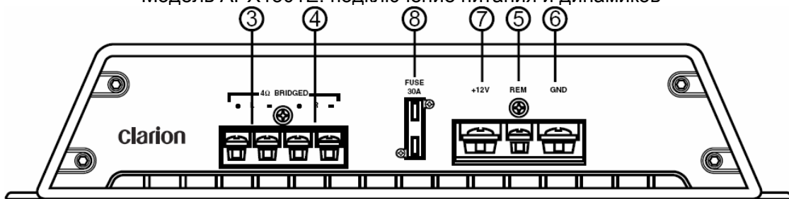
Модель APX2121E: подключение питания и динамиков
