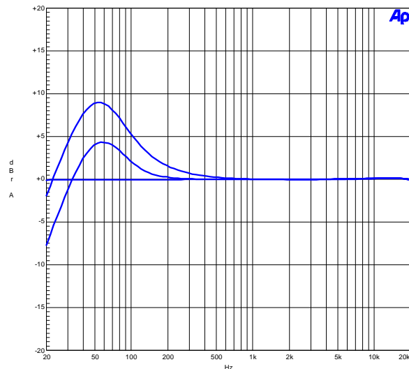
Abbildung 2-18: Frequenzgänge des LPN-Filters bei Einstellung High, Medium bzw. Flat.
