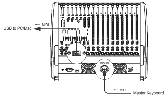
Abbildung 4-5: Übertragung von MIDI-Daten von einem Master Keyboard zum PC/Mac
