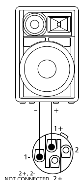
Abbildung 2-19: Anschlussbeispiel einer passiven Lautsprecherbox
