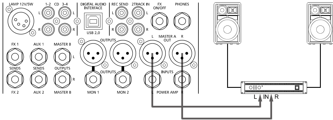
Abbildung 6-2: Anschluss eines externen Leistungsverstärkers an MASTER A OUT L/R
