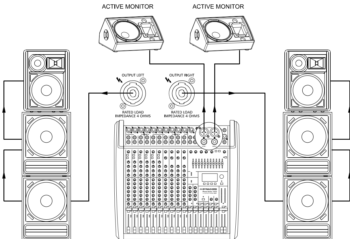
Abbildung 6-1: Maximale Ausbaustufe, Passivbetrieb
