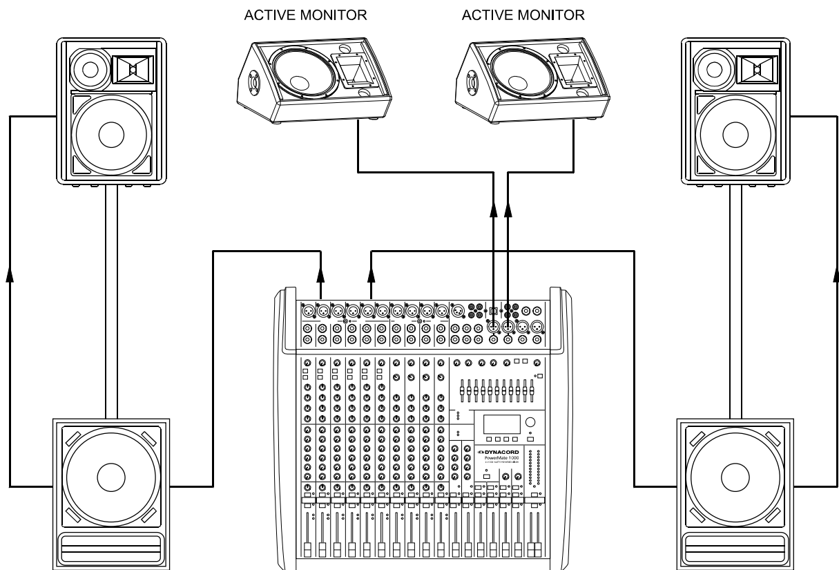
Abbildung 5-1: Aufbau einer Standard-PA
