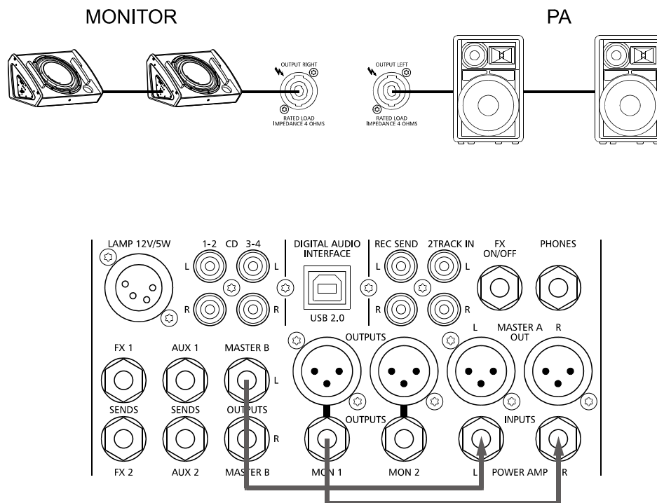
Abbildung 6-4: Mono PA + Monitor
