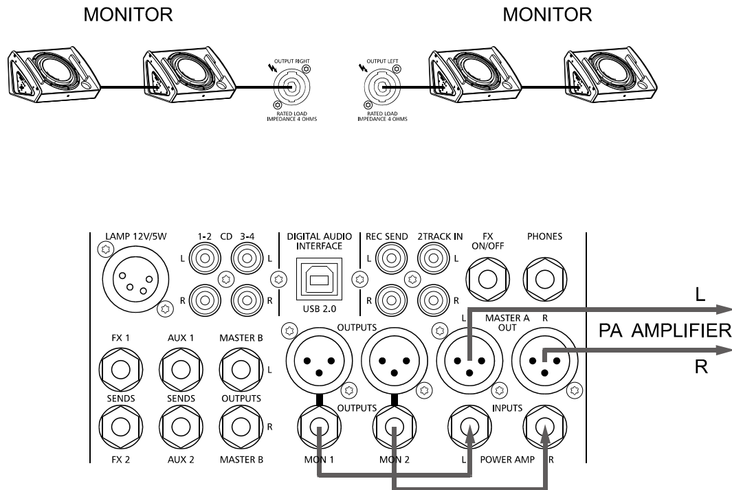
Abbildung 6-3: Verwendung der internen Endstufen für Monitore
