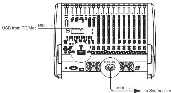
Abbildung 4-4: Übertragung von MIDI-Daten vom PC/Mac zu einem Synthesizer
