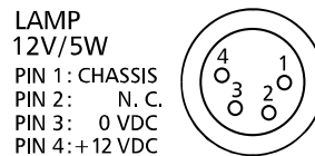
Abbildung 2-17: Belegung der LAMP 12V/5W-Buchse
