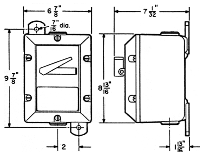
Figura 1 - Dimensiones
