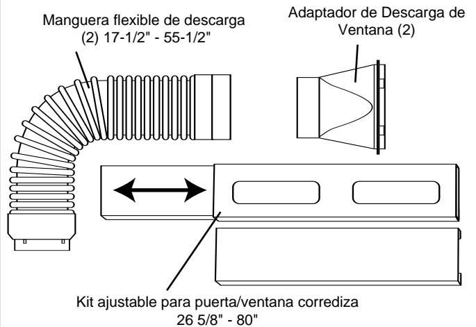
Fig. 1 a Accesorios del Tanque de Agua Externo
