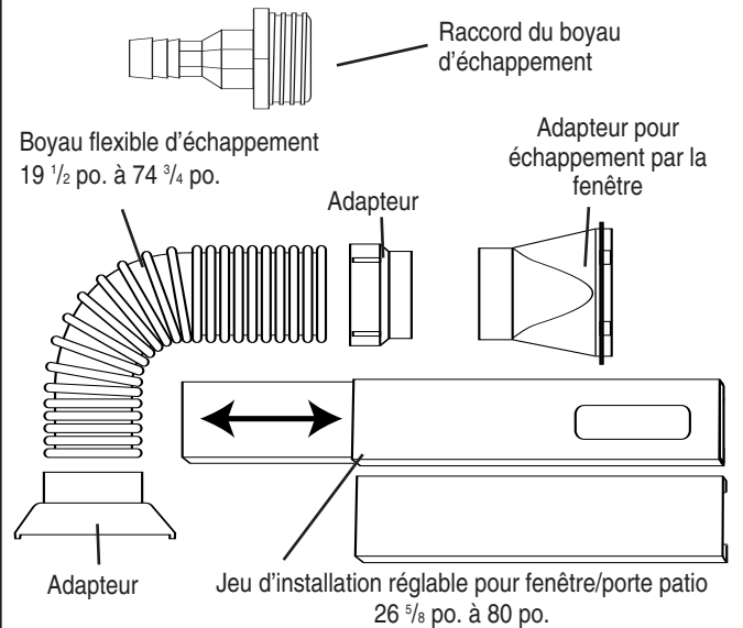
Fig. 1 Accessoires d'installation
