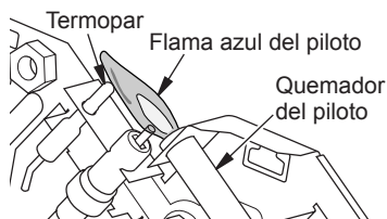
Figura 18 - Patrón correcto de la llama del piloto
