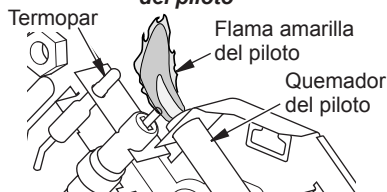
Figura 19 - Patrón incorrecto de la llama del piloto
