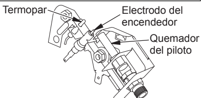
Figura 17 - Piloto
