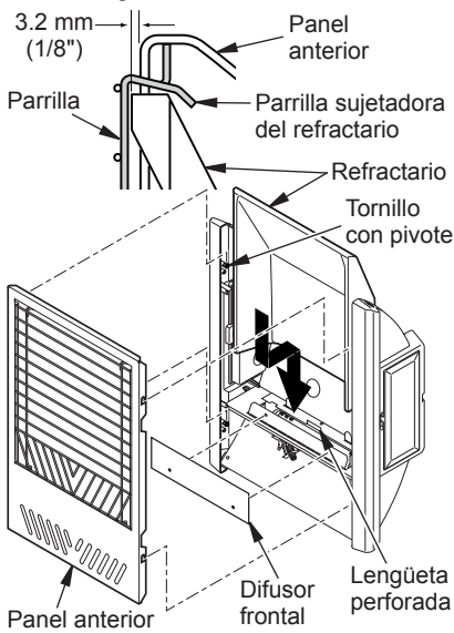
Figura 15 - Instalación del panel anterior y del refractario
