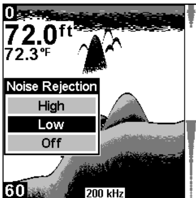
Noise Rejection menu.
