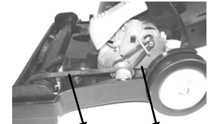
Fig. 52 Correa larga
