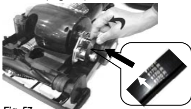
Correa corta
