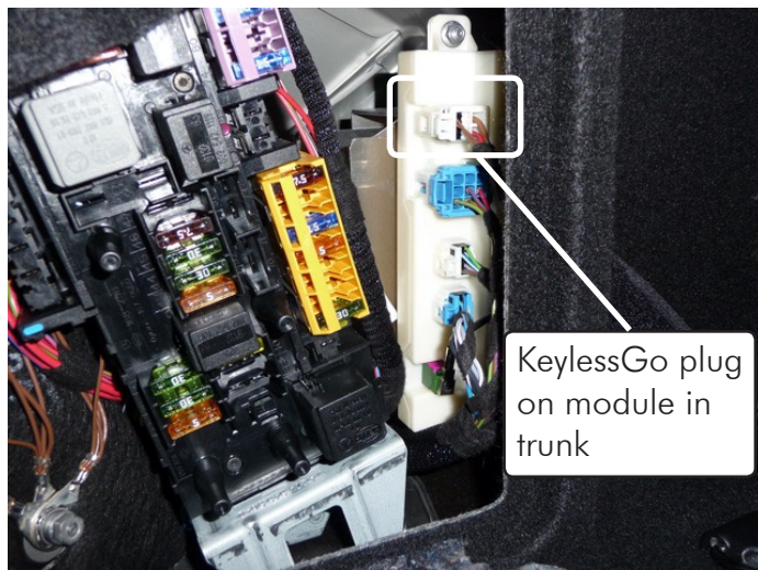
E coupe KeylessGo module -- right rear of trunk
