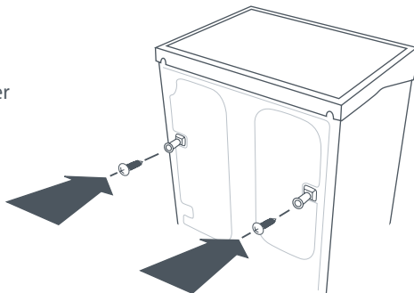
Fig. 10 Spacers
