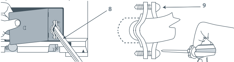
Dibujo 33 Regular el bloque terminal y los tornillos
