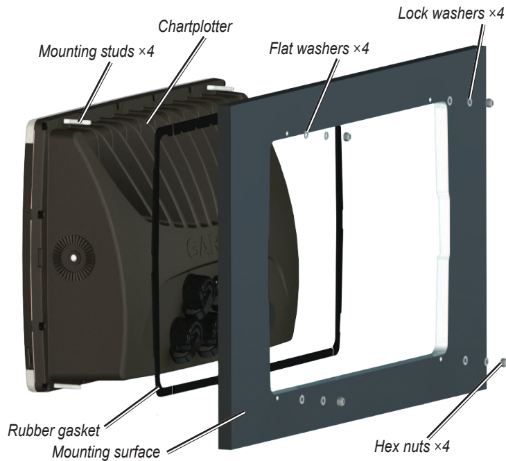
Flush Mounting a GPSMAP 4008/4208/4012/4212/5008/5208/5012/5212 Chartplotter
