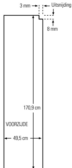
Paneel van koelgedeelte
