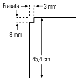
Pannello freezer senza distributore
