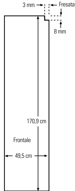
Pannello porta frigorifero
