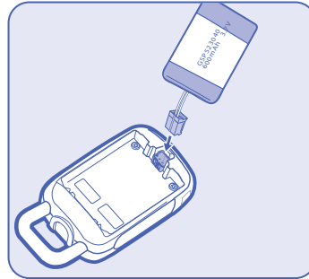
2 | Ponga la pila. Asegúrese de empujar apretadamente el conector.
