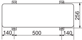
Dimensions de fixation au sol de l'unité extérieure (Unité: mm)
