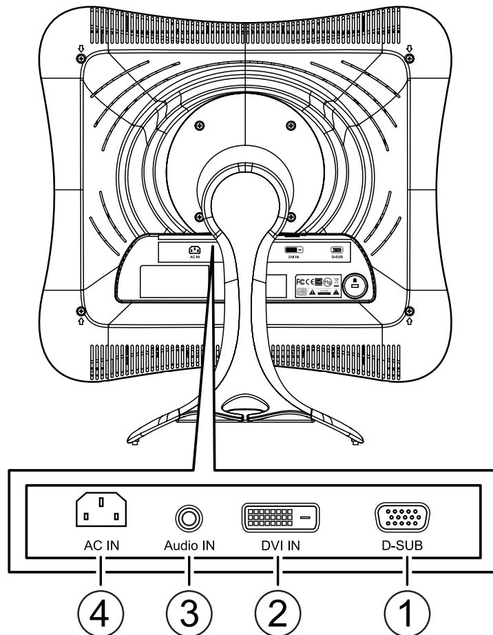
图二. 连接线
