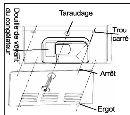
Ampoule du congélateur
