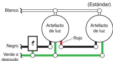
Esquema eléctrico 1
