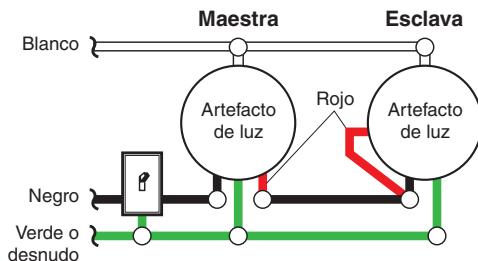
Esquema eléctrico 2
