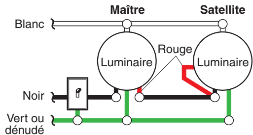
Diagramme de câblage 2
