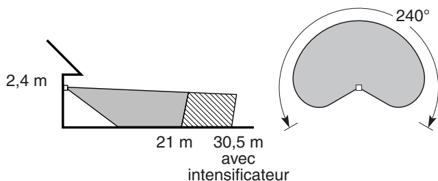
Portée maximale
