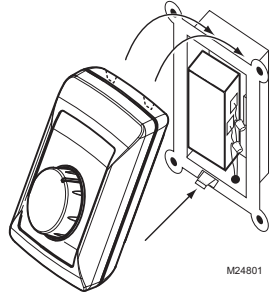
Fig. 11. Fixer l'humidistat sur la plaque de montage.
