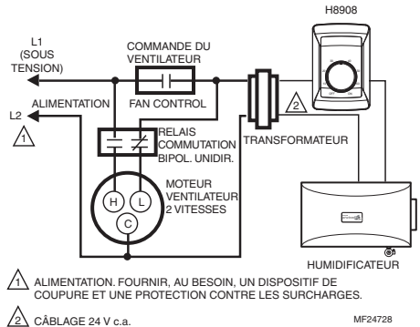
Fig. 13. Raccordement du H8908 avec un moteur de ventilateur à deux vitesses.
