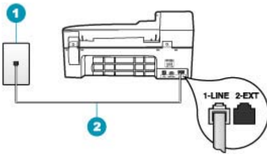
图 4-5 HP All-in-One 的后视图
