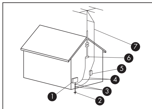
Mise à la terre de l'antenne
