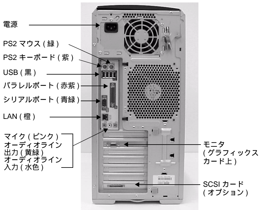
図 1-1 xw5000 背面パネルのコネクタ
