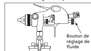
Figure 2 - Réglage sur le pistolet
